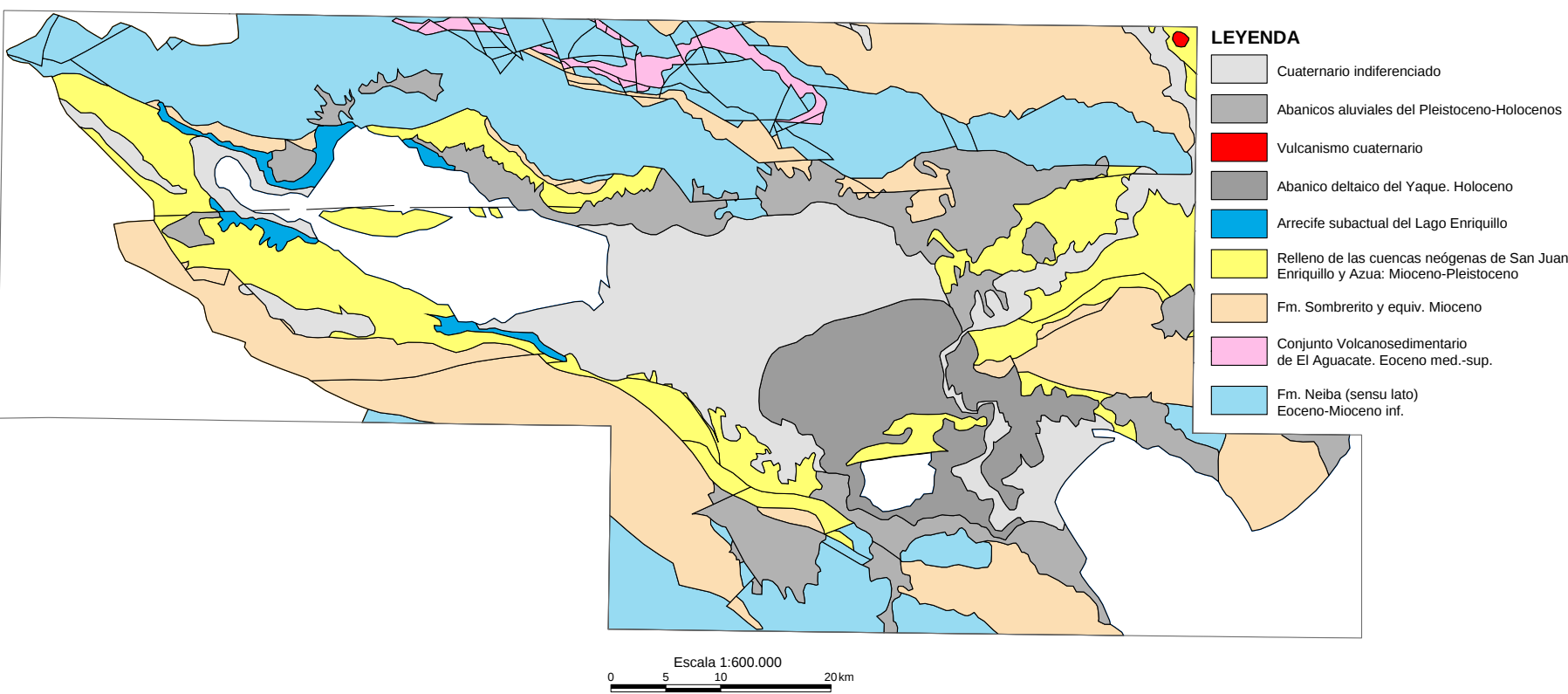
Esquema Geológico 1:600.000
