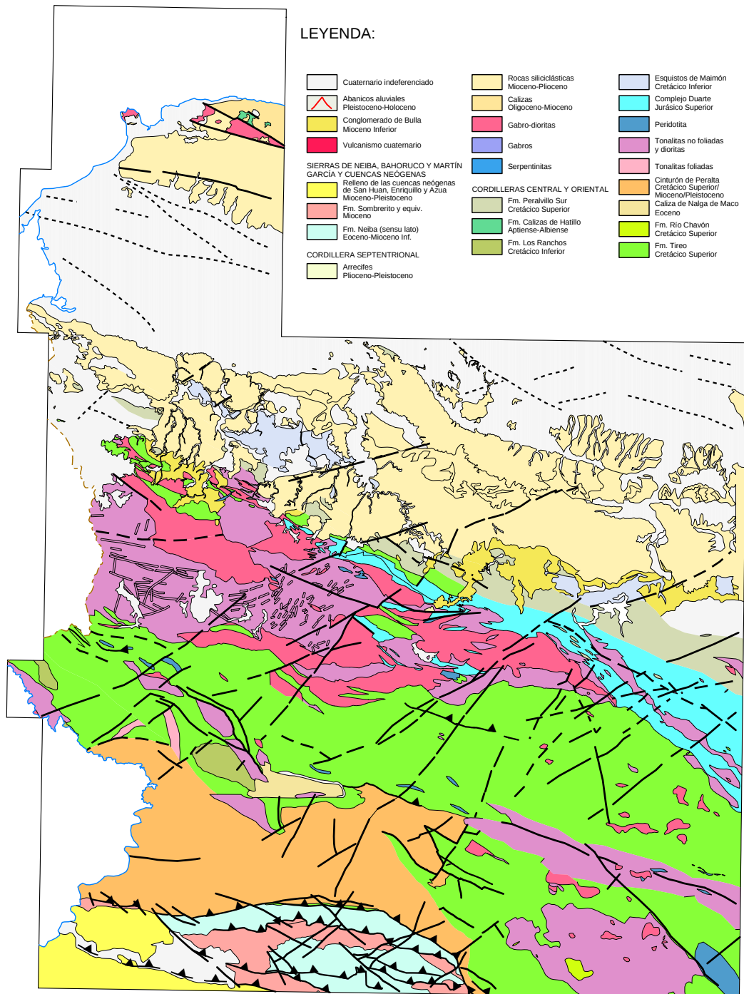
Esquema Geológico 1:600.000
