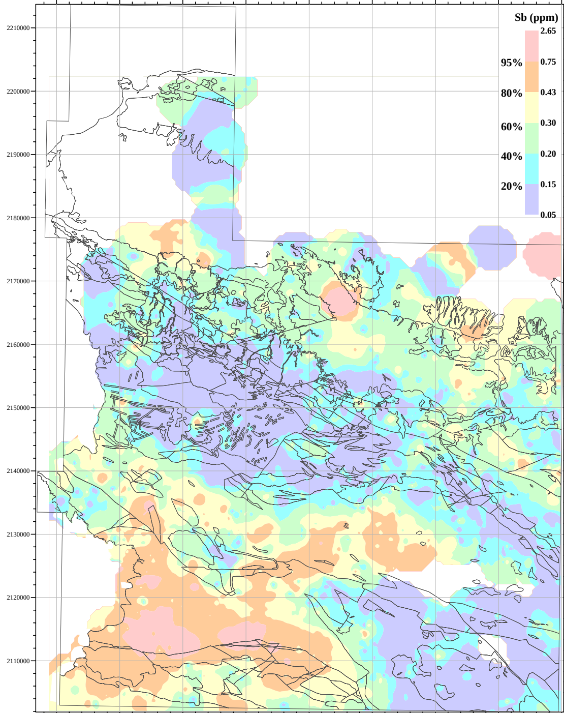
Mapa de distribución del Sb
