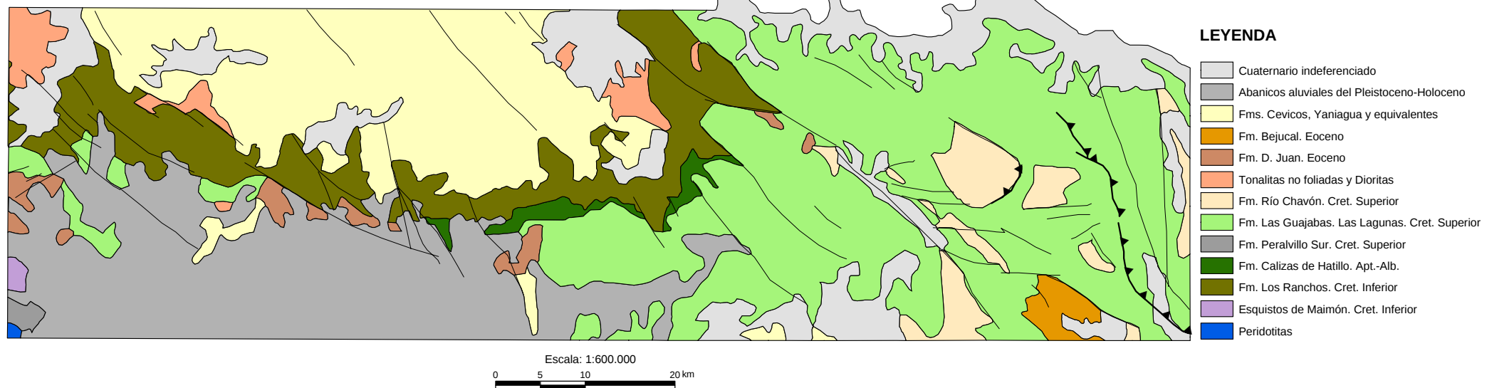
Esquema Geológico 1:600.000
