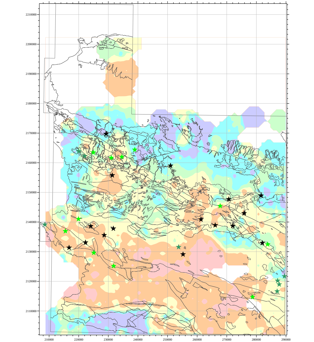
Mapa de distribución del índice de Hashimoto (MgO + K 2 O)/(MgO + K 2 O + CaO + Na 2 O)
