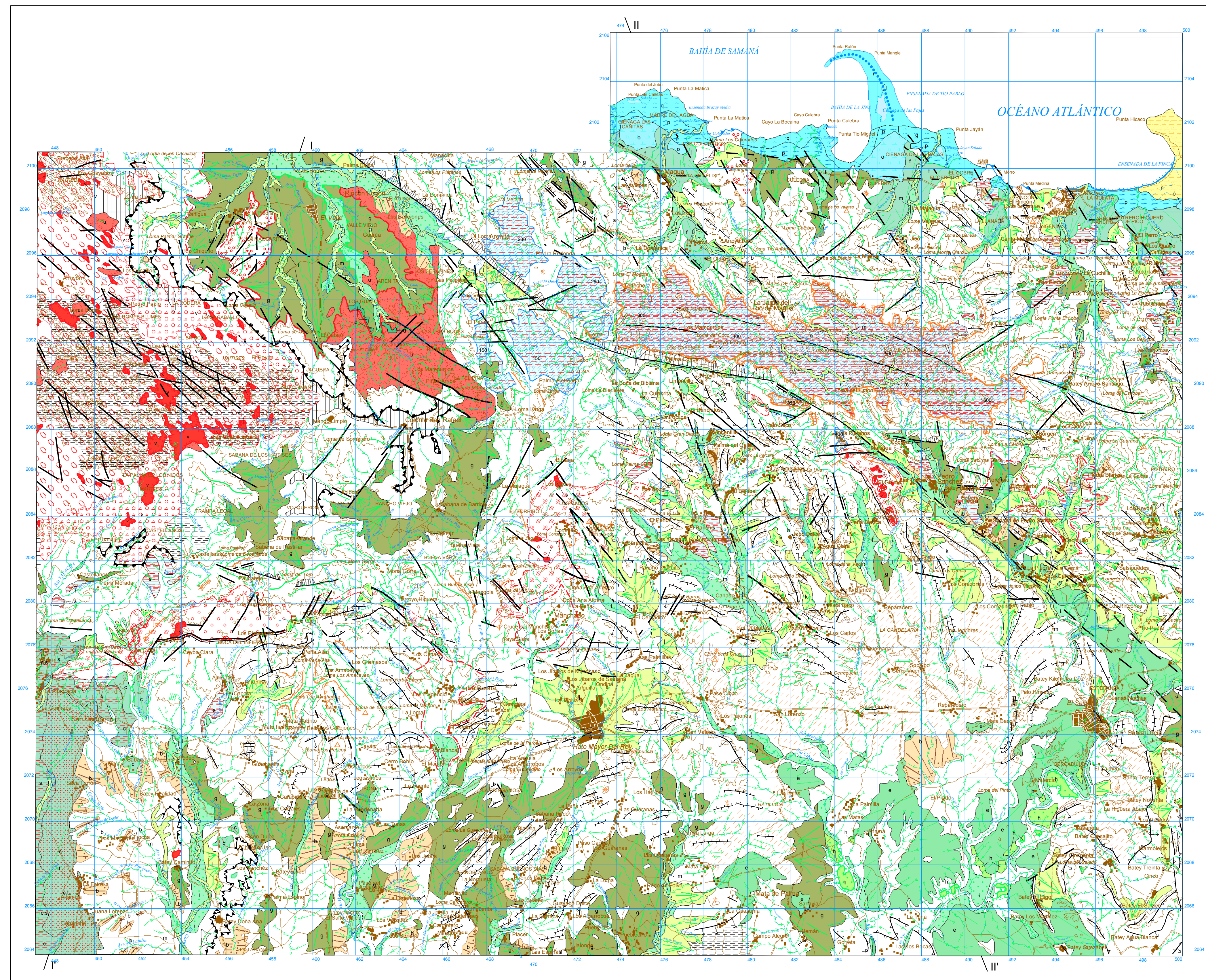
MAPA GEOMORFOLÓGICO DE LA REPÚBLICA DOMINICANA ESCALA 1:100.000
